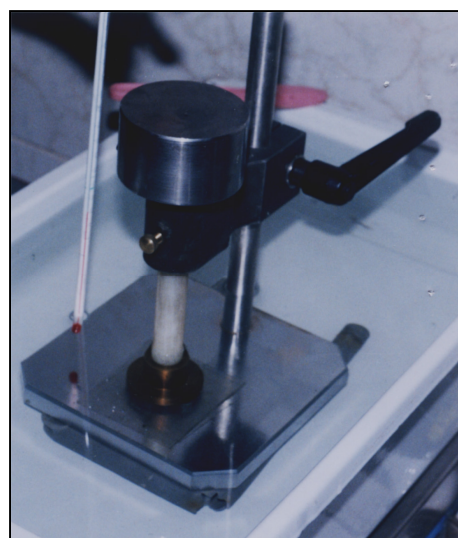
تصویر ۱- وسایل و نمونه در داخل هیتر، مربوط به تست سیلان موم Base Plate
