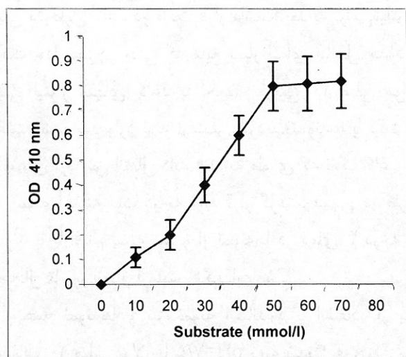
تصویر ۱- منحنی استاندارد اندازه‌گیری فعالیت آنزیم الاستاز مایع شیار لته‌ای
