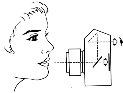
شکل ۲- دوربینهای تک لنز انعکاسی (SLR) که مشکل اختلاف منظر را ندارند
