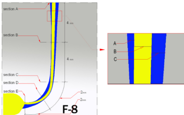
شکل ۵- پنج مقطع مورد بررسی تغییرات آناتومی کانالها
