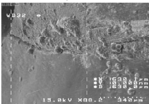
ب (۲)- تصویر FE-SEM از نمونه‌های ترمیم شده با گرانادیو در حالت اعمال سیکل مکانیکی
