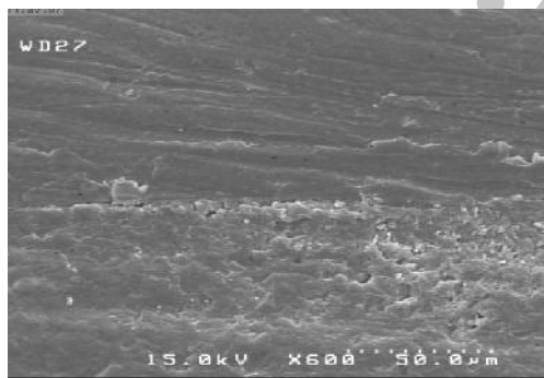
ب (۱)- تصویر FE-SEM از نمونه‌های ترمیم شده با گرانادیو
