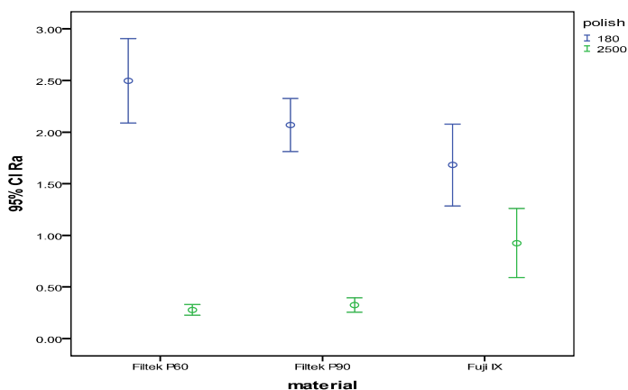
نمودار 1- مقایسه میانگین R_a مواد در 180 و 2500 grit
