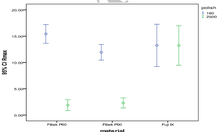
نمودار 2- مقایسه میانگین R_{max} مواد در 180 و 2500 grit
