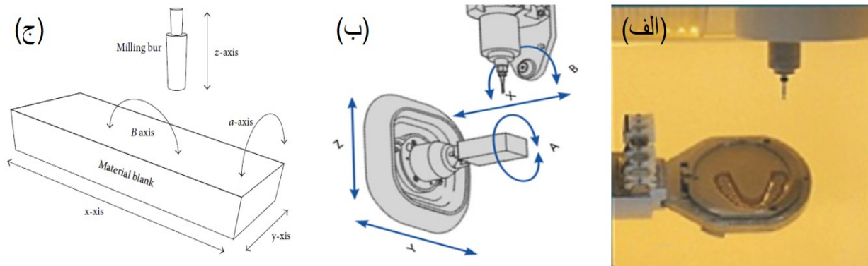
شکل ۸- محورها و اجزای اصلی ماشین فرز را نشان می‌دهد. (الف) نمایش اجزای ماشین فرز کنترل عددی دندانی (ب) و (ج) نمایش محورهای ماشین فرز (۸،۳۶).
