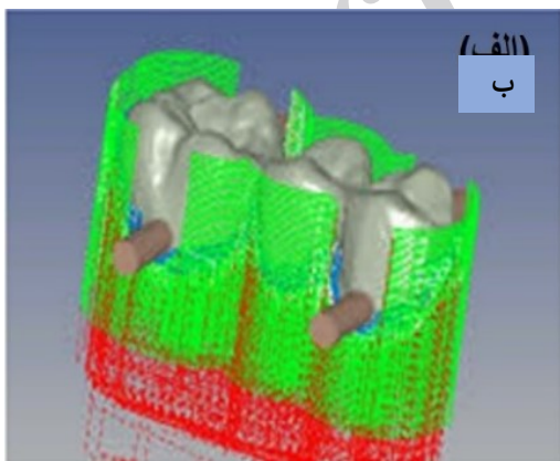
شکل ۷- برنامه ریزی تولید از طریق نرم افزار طرح ریزی را نشان می دهد. (الف) مسیر ابزار جهت تراش رستوریشن (ب) برنامه کنترل عددی (۳۵).
