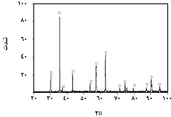
شکل ۵ - ج - الگوهای پراش پرتو X پودر کلسینه شده در ۱۰۰۰ درجه سانتی‌گراد به مدت ۱ ساعت ( \circ = \text{NiFe}_2\text{O}_4 ).
