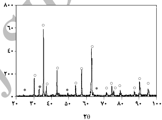
شکل ۵ - ب - الگوهای پراش پرتو X خاکستر حاصل از احتراق ( \circ = \text{NiFe}_2\text{O}_4 و * = \text{Fe}_2\text{O}_3 ).
