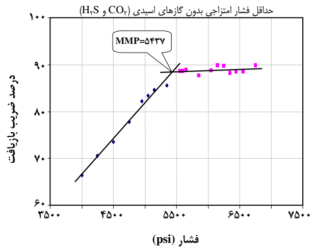
شکل ۲۳- نمودار فشار ضریب بازیافت نهایی، زمانی که درصد مولی H_2S و CO_2 به صفر ۰/۰ رسانده شده است.
