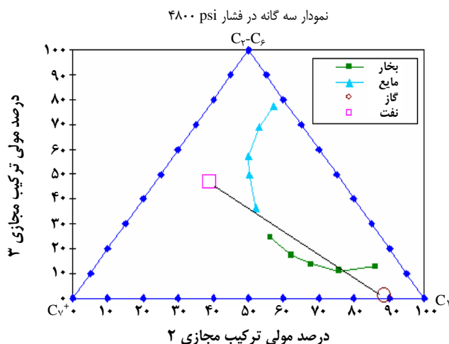
شکل ۱۶- نمودار سه فازي مربوط به فازهای ۶، ۷ و ۸ میدان گازی پارس جنوبی در فشار ۴۸۰۰ psi.
