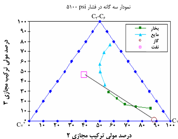
شکل ۱۷- نمودار سه فازي مربوط به فازهای ۶، ۷ و ۸ میدان گازی پارس جنوبی در فشار ۵۱۰۰ psi.
