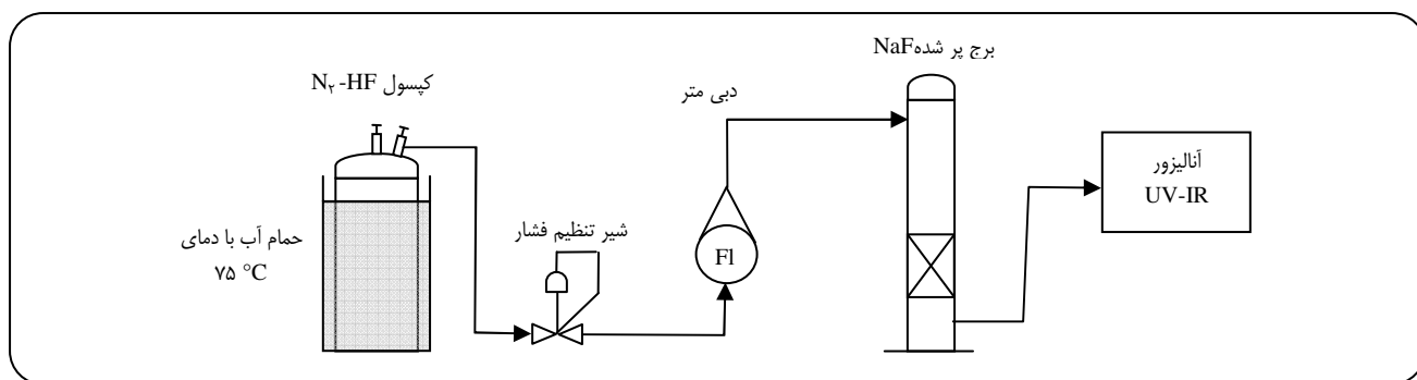
شکل ۴- شمای قرار گیری تجهیزات و نحوه اتصال آنها.
