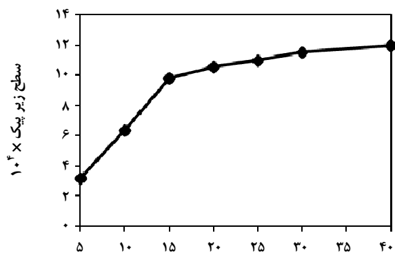
شکل ۵- اثر زمان استخراج بر کارایی استخراج نسبی آنالیت.
