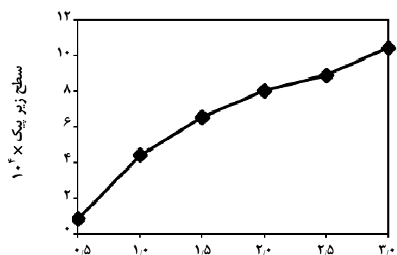
شکل ۶- اثر حجم قطره آلی بر کارایی استخراج نسبی آنالیت.
