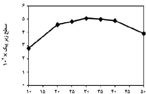
شکل ۷- اثر دمای محلول نمونه آبی (فاز دهنده) بر کارایی استخراج نسبی آنالیت.
