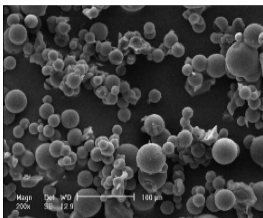
شکل ۱۱- تصویر SEM ذرات SAMPS ( نمونه ۱) با بزرگ نمای ۲۰۰ برابر.
