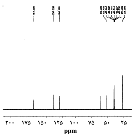
شکل ۷ - طیف ^{13}\text{C-NMR} مربوط به نمونه ۲.
