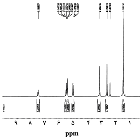
شکل ۸ - طیف ^1\text{H-NMR} مربوط به نمونه ۱.
