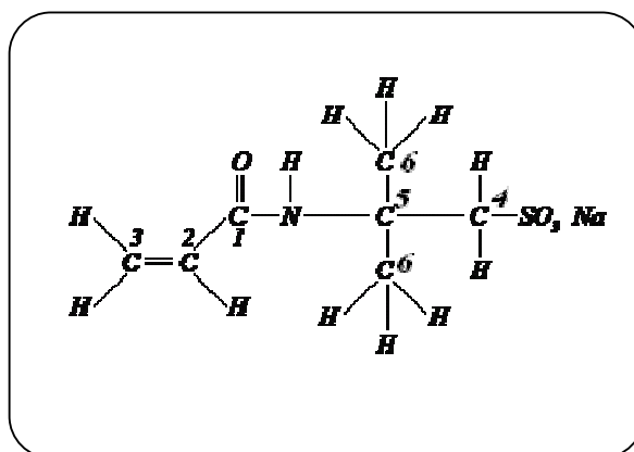
شمای ۲ - شماره گذاری کربن های موجود در ساختار SAMPS به منظور تحلیل طیف های ^{13}\text{C-NMR} .
