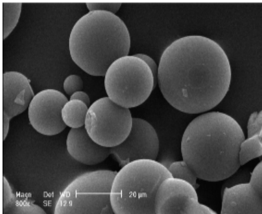
شکل ۱۲- تصویر SEM ذرات SAMPS ( نمونه ۱) با بزرگ نمای ۸۰۰ برابر.
