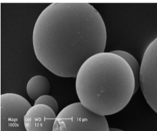
شکل ۱۳- تصویر SEM ذرات SAMPS ( نمونه ۱) با بزرگ نمای ۱۶۰۰ برابر.
