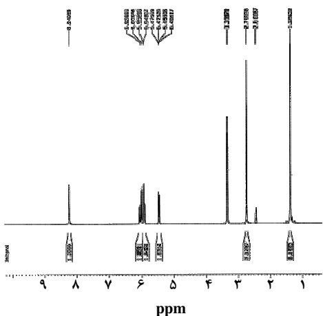
شکل ۹ - طیف ^1\text{H-NMR} مربوط به نمونه ۲.
