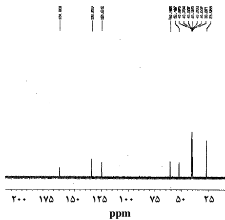
شکل ۶ - طیف ^{13}\text{C-NMR} مربوط به نمونه ۱.
