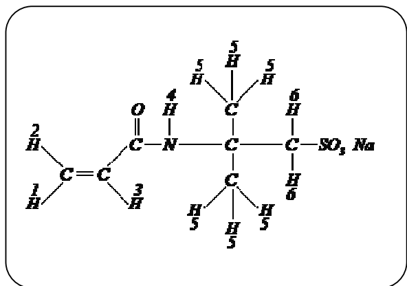
شمای ۳ - شماره گذاری هیدروژن های موجود در ساختار SAMPS به منظور تحلیل طیف های ^1\text{H-NMR} .
