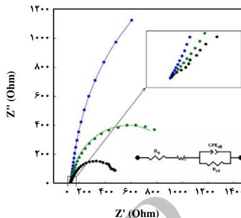
شکل ۲۲- نمودارهای نایکوئیست نانوپوسته‌های کبات اکسید در پتانسیل‌های ۵۷۰، ۶۱۰، ۶۵۰ mV مدار معادل الکتریکی و نمودارهای نایکوئیست شبیه‌سازی شده.
