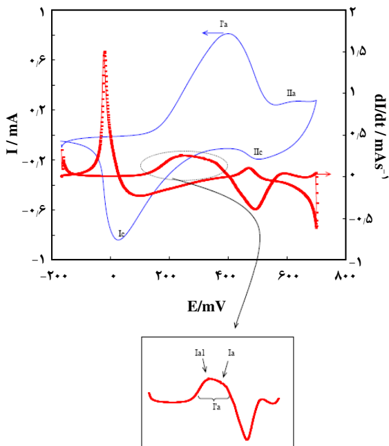
شکل ۹- ولتاموگرام چرخه ای و فرم مشتقی این ولتاموگرام برای الکتروپوشیده شده با نانوپوشته های کبالت اکسید (II) در محلول سدیم هیدروکسید ۱۰۰ mM با سرعت روبش ۵۰ mV/s.
