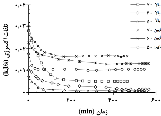
شکل ۴- اثر دما بر تلفات و بازده اکسرژی دو طبقه بستر سیال و بستر ثابت.
