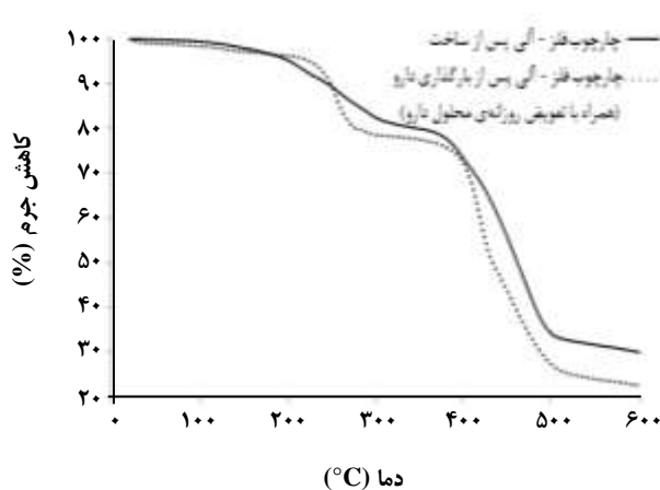
شکل ۳- آزمایش وزن سنجی گرمایی نمونه‌ها.
