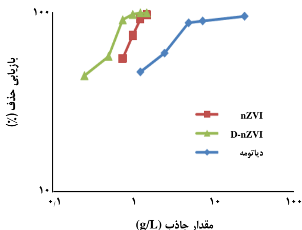
شکل ۶- بازیابی حذف نسبت به مقدار جاذب‌های nZVI و D-nZVI و دیاتومه.
