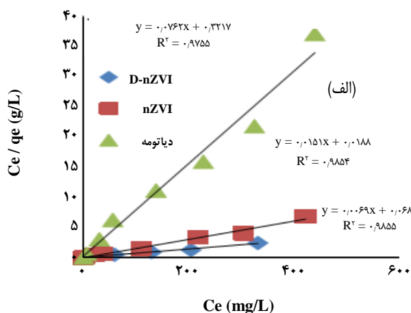
شکل ۷ - ایزوترم جذب فلز نیکل بوسیله سه جاذب nZVI و D-nZVI و دیاتومه.
