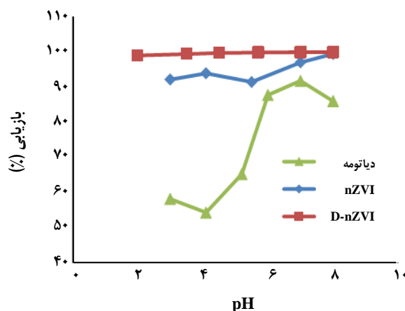
شکل ۵- تأثیر pH در جذب یون‌های نیکل توسط سه جاذب nZVI، D-nZVI و دیاتومه.
