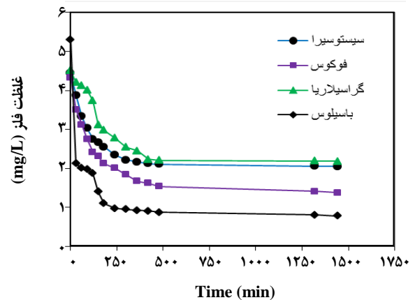
شکل ۲- بررسی سینتیکی جذب یون نیکل به‌وسیله جاذب‌ها. ( شرایط آزمایش: دمای ۲۵ درجه سلسیوس، میزان جاذب ۱ گرم بر لیتر، غلظت فلز ۴ میلی گرم بر لیتر، pH حدود ۶).
