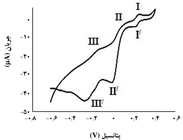
شکل ۶ - ولتاگرام چرخه‌ای ترکیب ۱.
