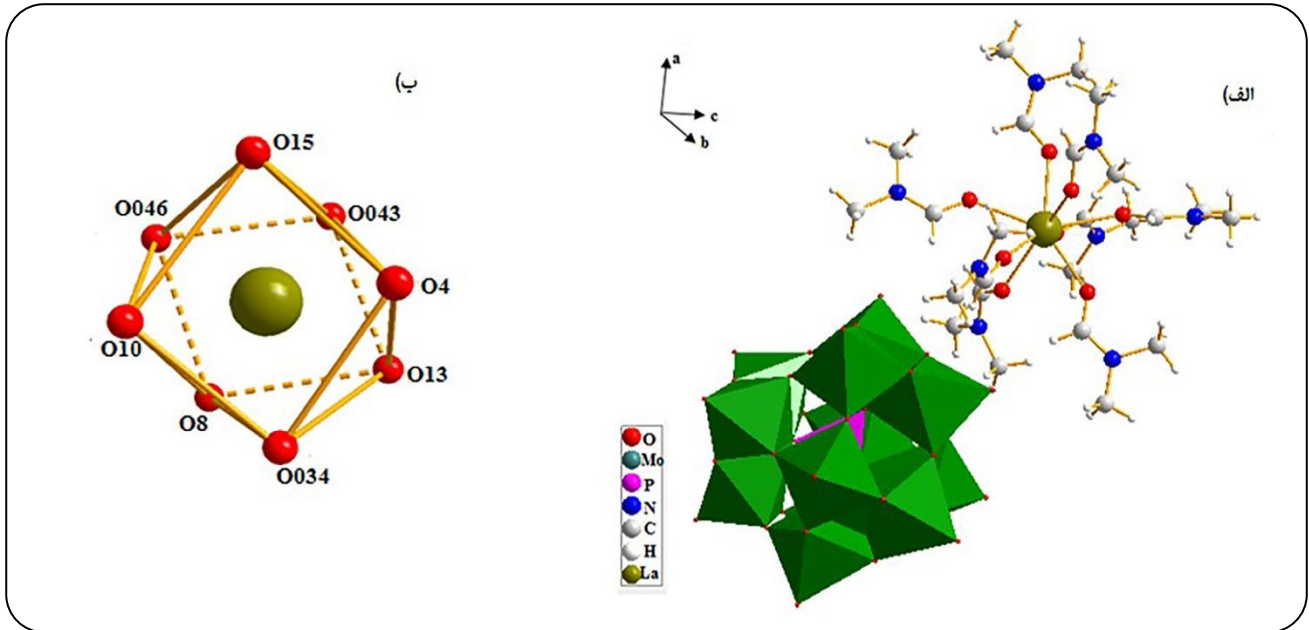
شکل ۵ - نمایش ساختار دو بُعدی ترکیب ۱ در راستای صفحه‌ی (۲۰۱).
