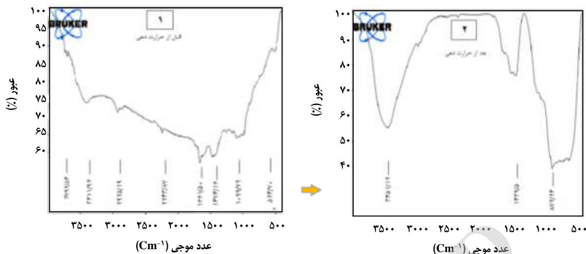
شکل ۴- طیف فرسرخ (FT-IR) نانوالیاف تهیه شده به روش الکتروریسی (۱): نانو الیاف شامل پیش ماده سرامیکی و پلیمر پیش از عملیات گرمایی، (۲): نانوالیاف سرامیکی پس از عملیات گرمایی.
