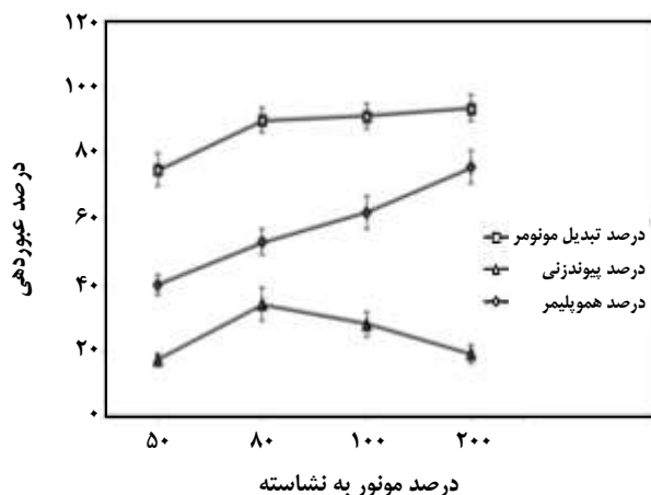
شکل ۴- اثر نسبت وزنی مونومر بر پارامترهای پیوند زنی (نسبت وزنی آغازگر به نشاسته ۲/۵٪، دما ۷۵ °C، زمان واکنش ۳ ساعت).
