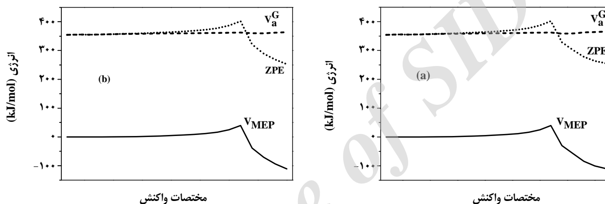
شکل ۶ - منحنی تغییرهای انرژی پتانسیل (MEP)، انرژی پتانسیل آدیباتیک حالت پایه ( V_a^G ) و انرژی نقطه‌ی صفر (ZPE) برای مسیر R1 (a) و R2 (b).
