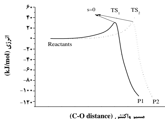
شکل ۳- منحنی انرژی پتانسیل برای واکنشهای R1 (خط پر)، R2 (نقطه چین)، که در سطح MP2/6-311++G(d,p) محاسبه شده است.
