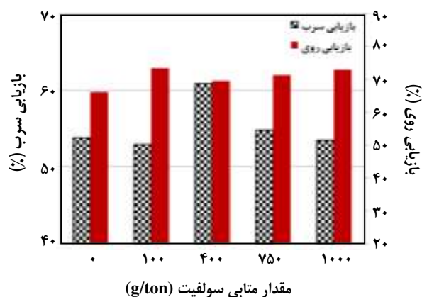
شکل ۵ - نمودار بازیابی سرب و روی در مقدارهای گوناگون متابی سولفیت.
