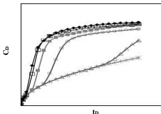
شکل ۱۳- تأثیر نسبت غیر همسانگردی kv/kh بر مقدار انحلال کربن‌دی‌اکسید در یک سامانه همگن - غیرهمسانگرد.
