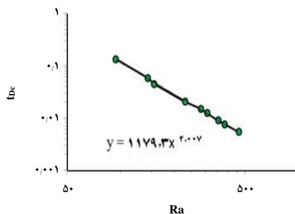
شکل ۱۰ - آغاز جابه‌جایی بر حسب تابعی از عدد رایلی با استفاده از شبیه‌سازی عددی.
