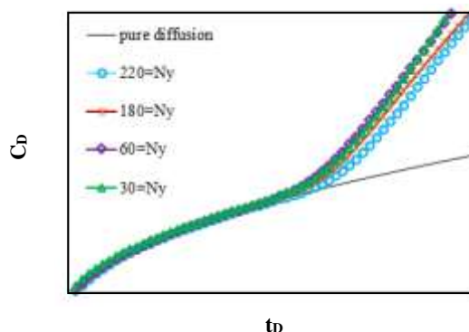
شکل ۶ - غلظت بدون بعد بر حسب زمان بدون بعد در اندازه شبکه‌های گوناگون (N_y = H/\Delta t) .
