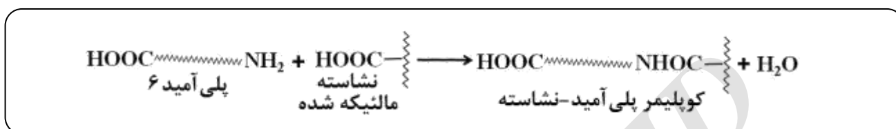
شمای ۲- واکنش بین گروه اسیدی و پلی آمید ۶.
