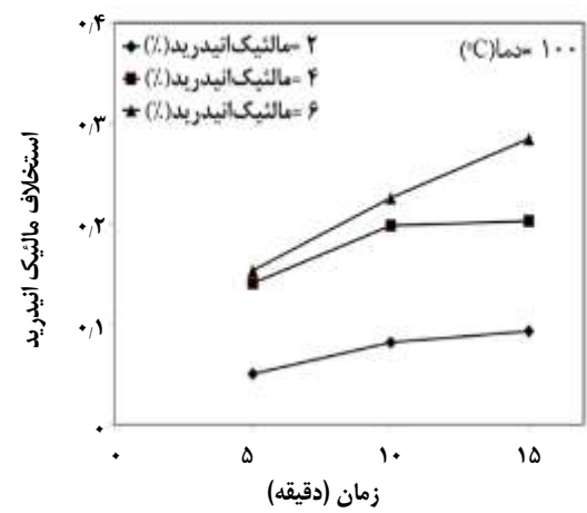
شکل ۱- میزان تغییر استخلاف مالیک آنیدرید بر اساس متغیرهای آزمایش.
