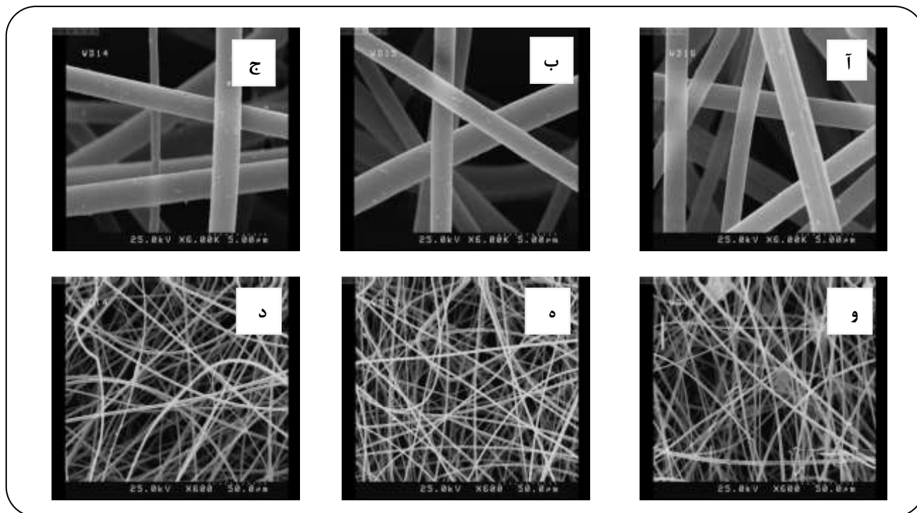
شکل ۳- عکس‌های SEM از بستر الیاف ریسیده شده در رطوبت نسبی ۵۰٪، مقدار نانو سیلیکا ۲ wt.% و دماهای (آ و د) ۲۵°C، (ب و ه) ۳۵°C و (ج و و) ۴۵°C در دو بزرگنمایی ۶۰۰ و ۶۰۰۰.
