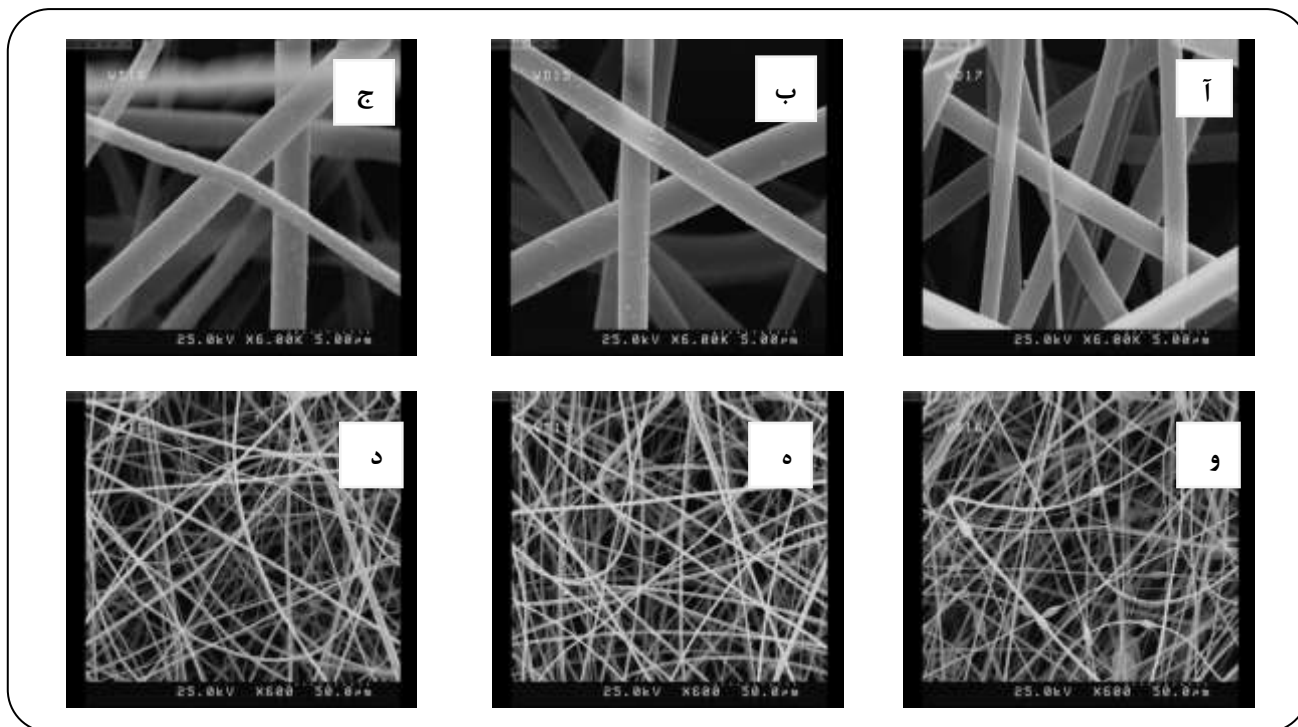
شکل ۴- عکس‌های SEM از بستر الیاف ریسیده شده در در رطوبت نسبی ۵۰٪ و دمای ۳۵°C و مقدارهای گوناگون نانو سیلیکا (آ و د) wt.٪ + ، (ب و ه) ۲ wt.٪ و (ج و و) ۴ wt.٪ در دو بزرگنمایی ۶۰۰ و ۶۰۰۰.
