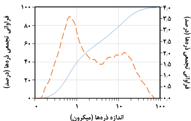
شکل ۲- نمودارهای توزیع دانه‌بندی (الف) هماتیت ریزدانه و (ب) هماتیت فوق ریزدانه. خط‌چین: نمودار فراوانی، خط ممتد: نمودار فراوانی تجمعی.
