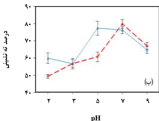
شکل ۶ - نمودار تاثیر متقابل (الف) بیوفلوکولانت- اندازه ذرات در pH ۷ و ۲% جامد و (ب) pH و اندازه ذرات در پلی ساکارید و ۵% جامد (○ فوق ریزدانه، Δ ریزدانه).
