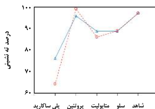
شکل ۶ - نمودار تاثیر متقابل (الف) بیوفلوکولانت- اندازه ذرات در pH ۷ و ۲% جامد و (ب) pH و اندازه ذرات در پلی ساکارید و ۵% جامد (○ فوق ریزدانه، Δ ریزدانه).
