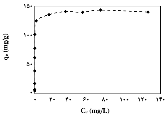
شکل ۳- ظرفیت جذب تعادلی بتونیت (q e ) بر حسب غلظت تعادلی متیلن‌بلو در محلول (C e ).
