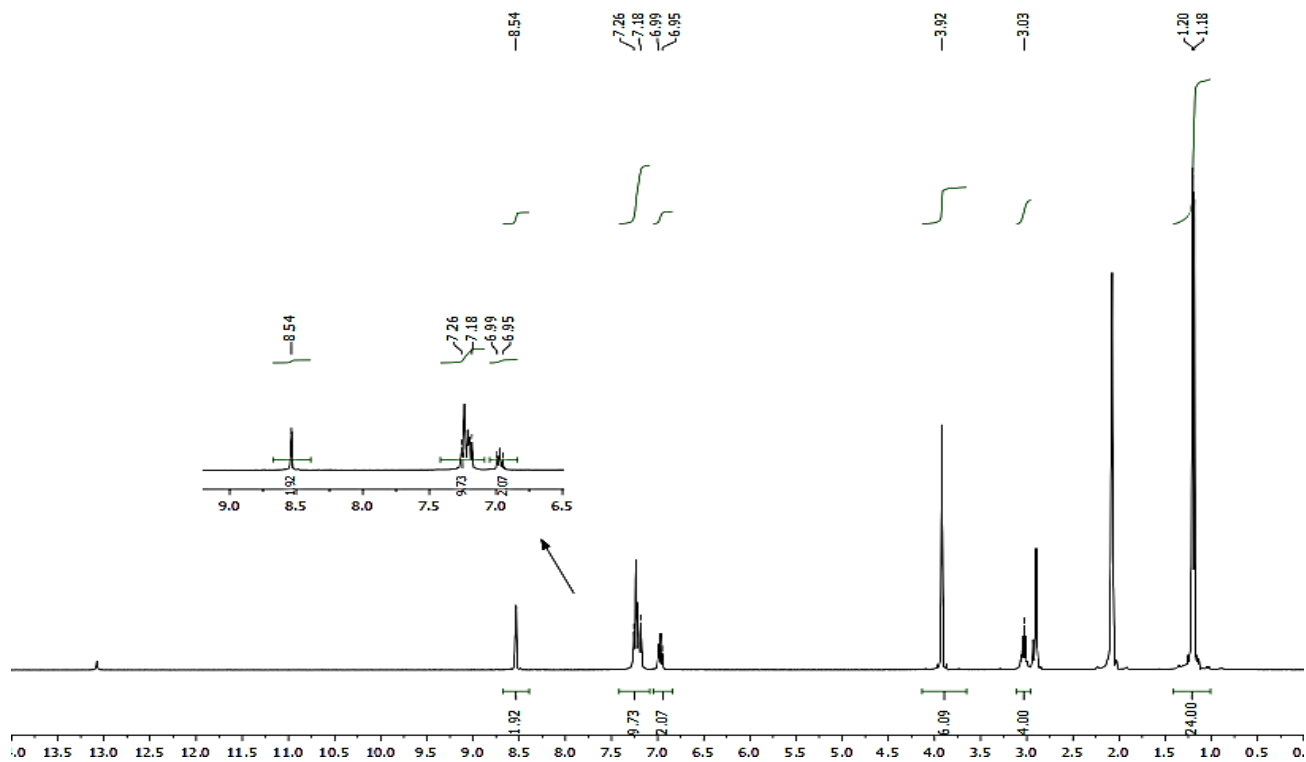
شکل ۶- طیف رزونانس مغناطیس هسته پروتون کمپلکس ۳
