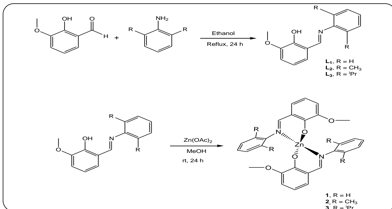
شماي ۲- مسیر سنتزی برای شیف بازهای L_1-L_3 و کمپلکس‌های فلز روی با این لیگاندها
