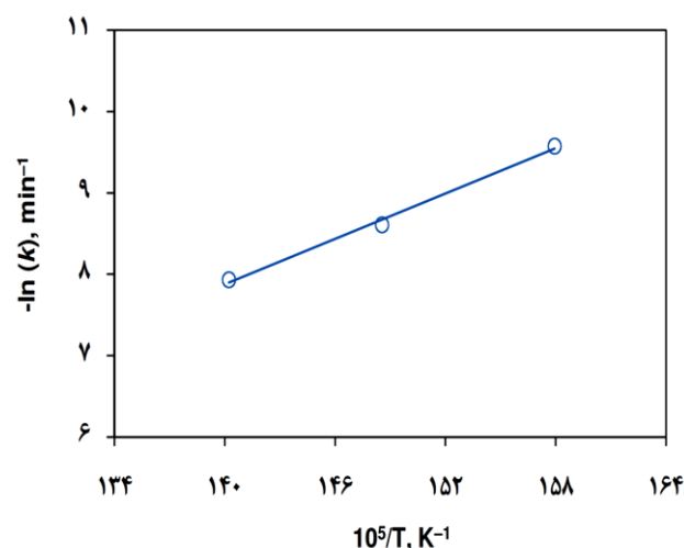
شکل ۲- نمودار آرنیوس منطبق شده بر داده‌های آزمایشگاهی در مرحله‌ی فراوری گرمایی در سه دمای گوناگون.
