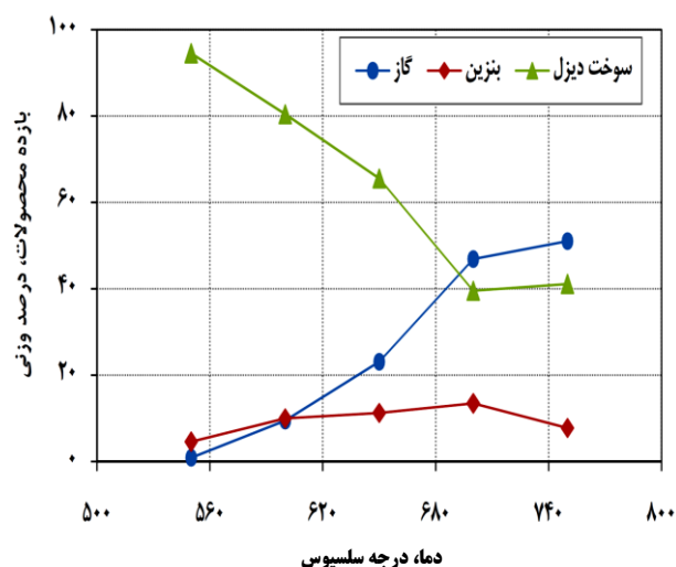
شکل ۶- بازده فراورده‌های به دست آمده از شکست گرمایی در دماهای گوناگون.
