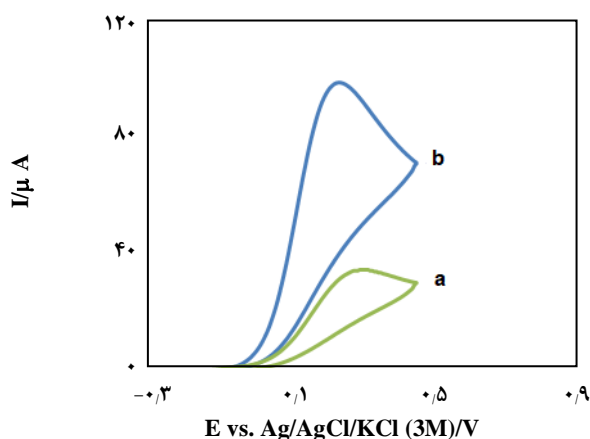
شکل ۲- ولتاموگرام های چرخه ای الکترودهای صفحه چاپی اصلاح نشده در محلول بافر فسفات ۰/۱ M (pH=۷/۰) (a) و الکترودهای صفحه چاپی اصلاح شده در محلول بافر فسفات ۰/۱ M (pH=۷/۰) (b). در هر دو حالت محلول دارای ۱۵۰/۰ μM دوپامین و سرعت روبش ۵۰ میلی ولت بر ثانیه بود.
