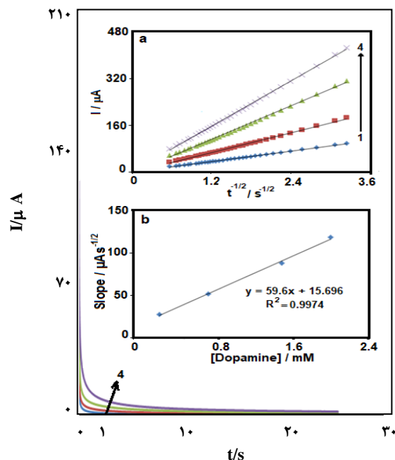
شکل ۵- کروئوآمپروگرام‌های متفاوت‌های غلظت‌های دوپامین در محلول بافر فسفات ۰/۱ M (pH=۷/۰) با پله پتانسیل ۳۵۰ میلی ولت. عدد‌های ۱ تا ۴ به ترتیب به غلظت‌های ۰/۳، ۰/۷، ۱/۵، و ۲/۰ میلی مولار مربوط هستند. پیوست‌ها (a) تغییرهای I - t^{-1/2} به دست آمده از کروئوآمپروگرام‌های ۱-۴ و (b) شیب خطوط I - t^{-1/2} بر حسب غلظت دوپامین.
