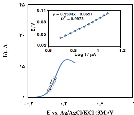
شکل ۴- ولتاموگرام روبش خطی ۱۵۰/۰ میکرومولار دوپامین در محلول بافر فسفات ۰/۱ M (pH=۷/۰) در سرعت روبش ۵ mV s -1 . ضمیمه: تغییرهای پتانسیل در مقابل لگاریتم جریان (نمودار تافل).
