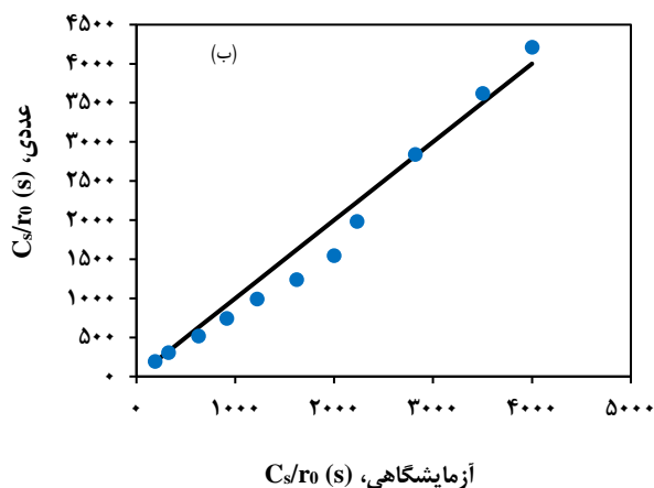
شکل ۱۲ - نمودار دوگانه مقایسه حل روش (الف) تقریب درجه سوم و (ب) حل عددی با داده های آزمایشگاهی.
