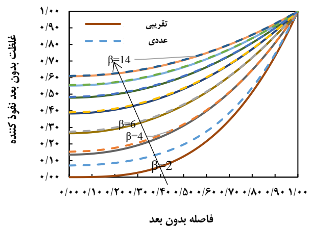
شکل ۳- مقایسه حل تقریب درجه سوم و حل عددی غلظت ماده نفوذ کننده بر حسب طول برای مقادیرهای \phi^2 = 4 و \beta = 2, 4, 6, 8, 10, 12, 14 .
