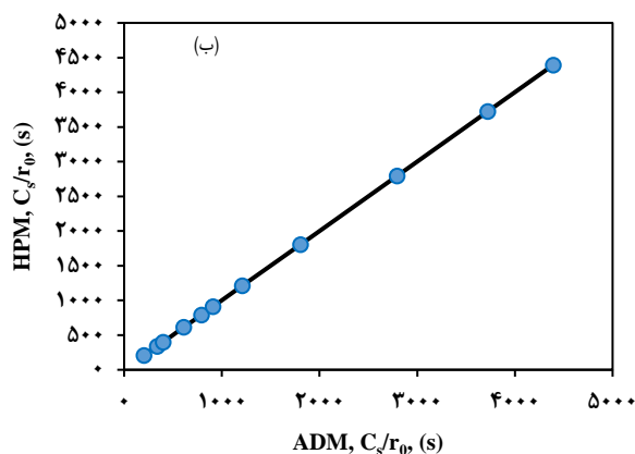
شکل ۱۱ - مقایسه روش هوموتوپی با (الف) داده های آزمایشگاهی و (ب) روش تجزیه آدومین در نمودارهای دوگانه.
