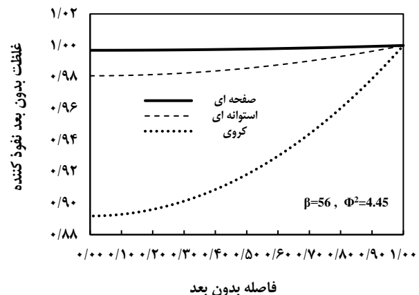
شکل ۱۰ - غلظت بی‌بعد ماده نفوذ کننده در امتداد طول بی‌بعد برای هندسه‌های گوناگون توسط روش HPM.
