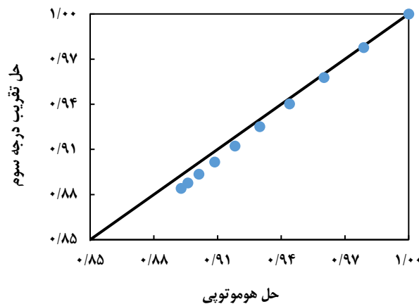
شکل ۸- مقایسه حل HPM و حل تقریب درجه سوم برای کاتالیست واقعی اول.
