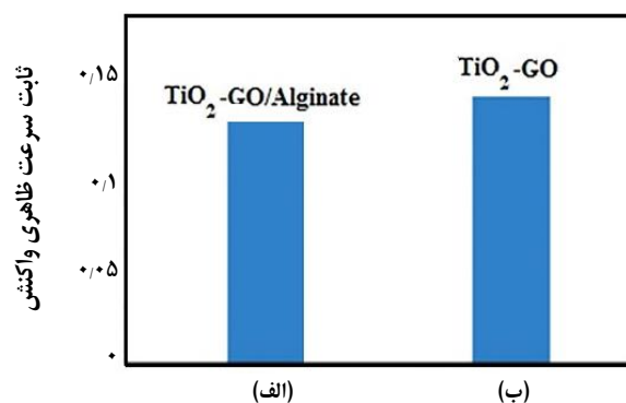
شکل ۸ - بررسی فعالیت فتوکاتالیزوری TiO_2 -Graphene و TiO_2 -Graphene/Alginate در حذف متیل اورانژ از محلول های آبی.
