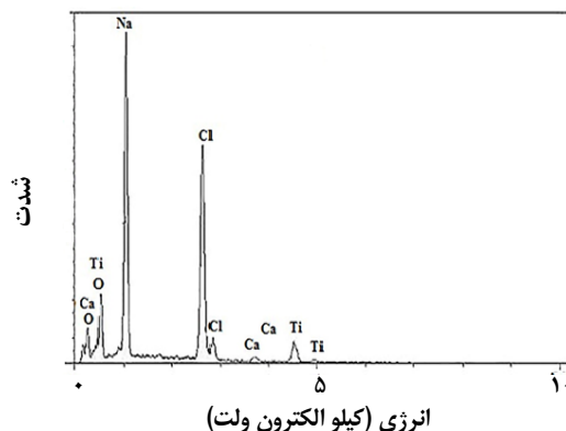
شکل ۴- آنالیز EDX نانوکامپوزیت TiO_2 - Graphene/Alginate.
