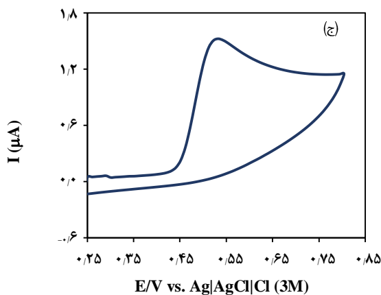
شکل ۳ - الف) ولتاموگرام های چرخه‌ای GCE، ERGO/GCE، Pt-ERGO/GCE، Pt-Pd/ERGO/GCE و Pt-ERGO/GCE در حضور BPA با \text{pH}=8 و در غیاب BPA (ب) در حضور BPA 0.1 \text{ mM} در سرعت روبش 50 \text{ mV/s} (ج) تصویر بزرگ شده منحنی مربوط به رفتار اکسایشی BPA بروی GCE می‌باشد.
