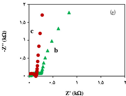
شکل ۲- الف) ولتاموگرام چرخه‌ای GCE(a)، ERGO/GCE(b) و Pt-Pd/ERGO/GCE (c) در محلول 0.1 M KCl دارای 1 mM K_3[Fe(CN)_6] با سرعت روبش 50 \text{ mV s}^{-1} (ب) نمودارهای نایکوئیست مربوط به GCE(a)، ERGO/GCE(b) و Pt-Pd/ERGO/GCE(c) در محلول 0.1 M از 1 mM حاوی Fe(CN)_6^{3-/4-} در پتانسیل مدار باز (ج) تصویر بزرگ شده نمودارهای نایکوئیست b و c می باشد.
