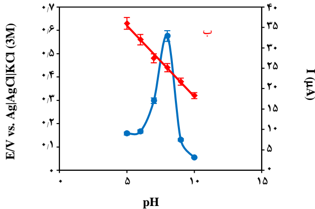
شکل ۷-الف) ولتاموگرام با روبش خطی در سطح Pt-Pd/ERGO/GCE در 0.1 M PBS با مقدار pH مختلف (a) ۵، (b) ۶، (c) ۷، (d) ۸، (e) ۹ و (f) ۱۰ در حضور 0.1 mM BPA با سرعت روبش 50 mV/s و (ب) نمودار تغییر پتانسیل (b) جریان بر حسب pH.
