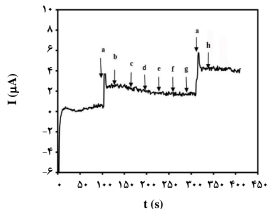
شکل ۱۰- آمپروگرام مربوط به Pt-Pd/ERGO/GCE با افزایش 5 \mu\text{M} از BPA در غیاب و حضور گونه‌های مزاحم با غلظت ۱۰۰ برابر (a) BPA، (b) گلوکز، (c) \text{Na}^+ ، (d) اوره، (e) \text{NO}_3^- ، (f) \text{NO}_2^- ، (g) \text{F}^- و (h) \text{CO}_3^{2-} .
