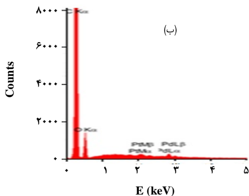
شکل ۱- الف ( FESEM و ب) نتیجه‌های آنالیز EDX مربوط به Pt-Pd/ERGO/GCE
