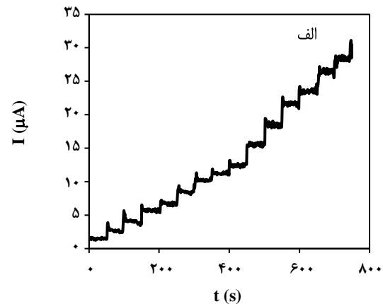
شکل ۹- الف) آمپروگرام مربوط به Pt-Pd/ERGO/GCE با افزایش ترکیب BPA در بازه غلظتی 5-201/5 \mu\text{M} و ب) منحنی درجه بندی جریان بر حسب غلظت.
