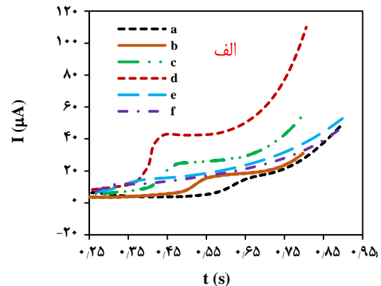
شکل ۷-الف) ولتاموگرام با روبش خطی در سطح Pt-Pd/ERGO/GCE در 0.1 M PBS با مقدار pH مختلف (a) ۵، (b) ۶، (c) ۷، (d) ۸، (e) ۹ و (f) ۱۰ در حضور 0.1 mM BPA با سرعت روبش 50 mV/s و (ب) نمودار تغییر پتانسیل (b) جریان بر حسب pH.
