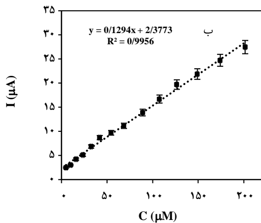
شکل ۹- الف) آمپروگرام مربوط به Pt-Pd/ERGO/GCE با افزایش ترکیب BPA در بازه غلظتی 5-201/5 \mu\text{M} و ب) منحنی درجه بندی جریان بر حسب غلظت.
