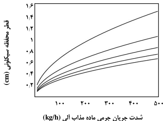
شکل ۵ - اثر شدت جریان جرمی ماده مذاب بر قطر مورد نیاز محفظه پاشی در دماهای گوناگون هوای خنک‌کننده.
