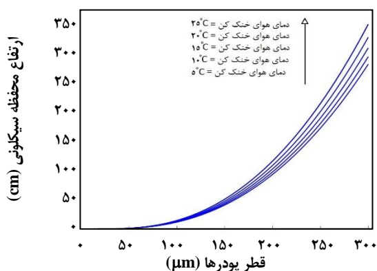
شکل ۴- اثر دمای هوای خنک کننده بر ارتفاع مورد نیاز سیکلون.
