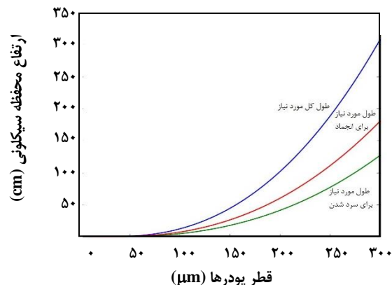
شکل ۳- تأثیر قطر پودر بر ارتفاع مورد نیاز برای محفظه پاششی.
