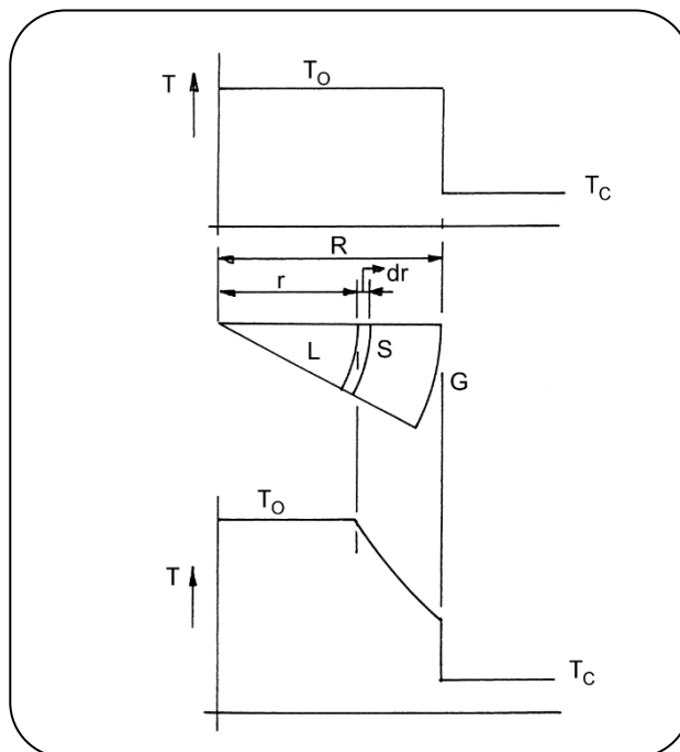
شکل ۲- پروفیل دمایی در درون قطره های کروی در حال انجماد.
