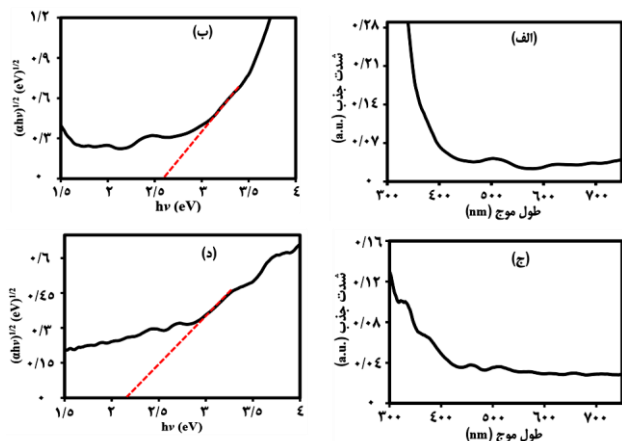
شکل ۵ - (الف) و (ج) طیف جذبی و (ب) و (د) تعیین گاف انرژی نمونه‌های ساخته شده با نسبت‌های بیسموت برابر با (الف) و (ب) ۰، (ج) و (د) ۱/۰.
