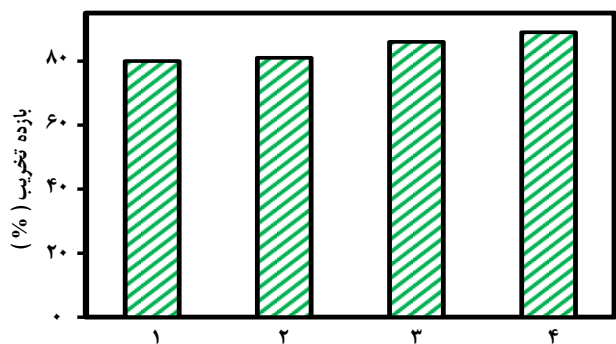
شکل ۸ - تکرار پذیری عملکرد کاتالیست نوری نمونه ساخته شده با نسبت بیسموت به تنگستن برابر با ۱/۰ تحت تابش لامپ زنون.
