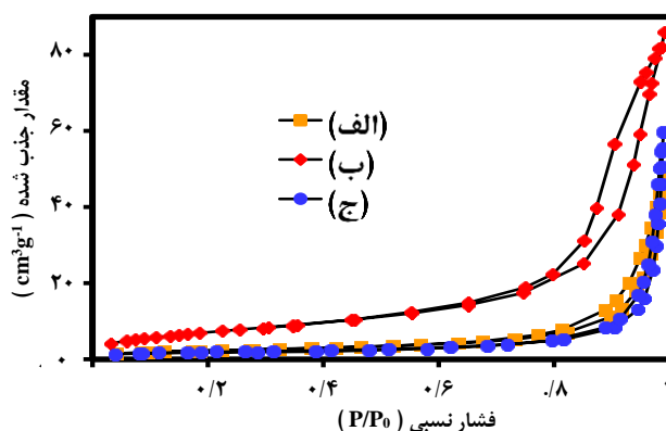
شکل ۴ - هم‌دمای جذب / واجذب گاز نیتروژن توسط نمونه‌های ساخته شده با نسبت‌های بیسموت به تنگستن برابر با (الف) ۰، (ب) ۱/۰، (ج) ۲/۰.
