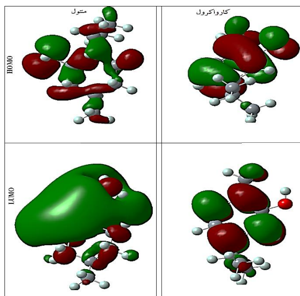
شکل ۲- اربیتال هومو و لومو دو ترکیب منتول و کارواکرول
