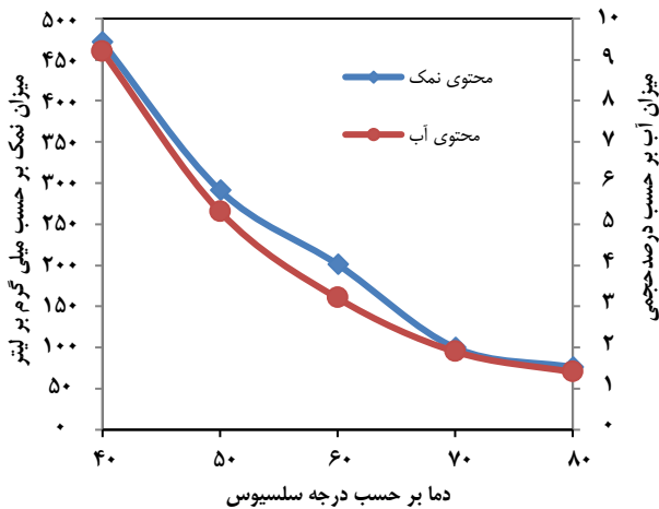
شکل ۹- میزان نمک نمونه نفت اهواز ۱ در دماهای گوناگون تزیق ۱۰ kHz و ۵٪ آب شست و شو و ۴۰ ppm تعلیق شکن تابش فراصوت با قدرت ۷۵ W و زمان ۶۰ دقیقه
