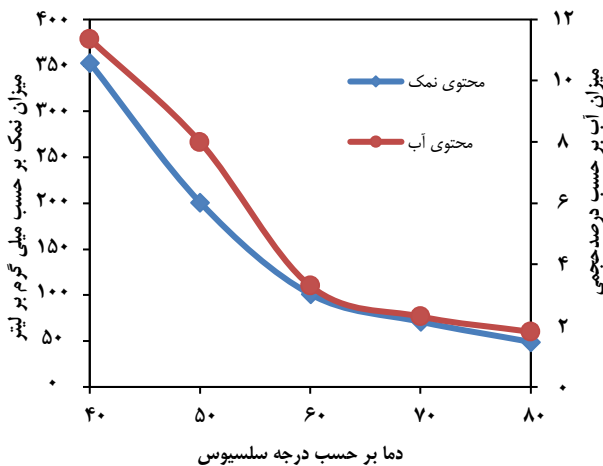
شکل ۱۰- میزان نمک نمونه نفت اهواز ۴ در دماهای گوناگون تزیق ۱۰ kHz و ۵٪ آب شست و شو و ۳۰ ppm تعلیق شکن تابش فراصوت با قدرت ۷۵ W و زمان ۶۰ دقیقه
