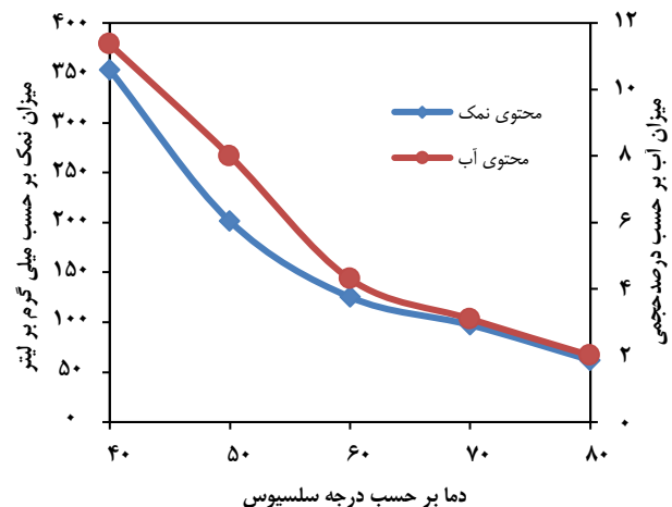
شکل ۸- میزان نمک نمونه نفت اهواز ۴ در دماهای گوناگون تزیق ۲۰ kHz و ۵٪ آب شست و شو و ۳۰ ppm تعلیق شکن تابش فراصوت با قدرت ۷۵ W و زمان ۶۰ دقیقه
