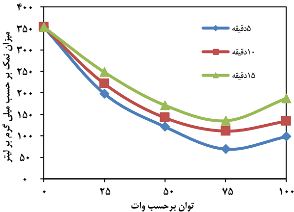
شکل ۱۱- میزان نمک اهواز ۴ با توان‌های ورودی متفاوت با زمان‌های تابش (۵ و ۱۰ و ۱۵ دقیقه) در میدان موج ایستاده با فرکانس ۲۰ kHz، زمان ته نشینی ۶۰ دقیقه و تزریق ۵٪ آب شست و شو و ۳۰ ppm تعلیق شکن در دمای ۸۰ درجه سلسیوس
