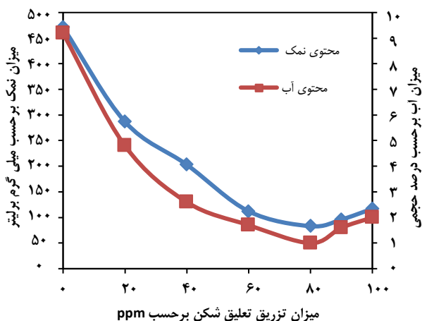
شکل ۱- تأثیر تزریق تعلیق شکن بر نمک‌زدایی و آب‌زدایی از نمونه نفت اهواز ۱
