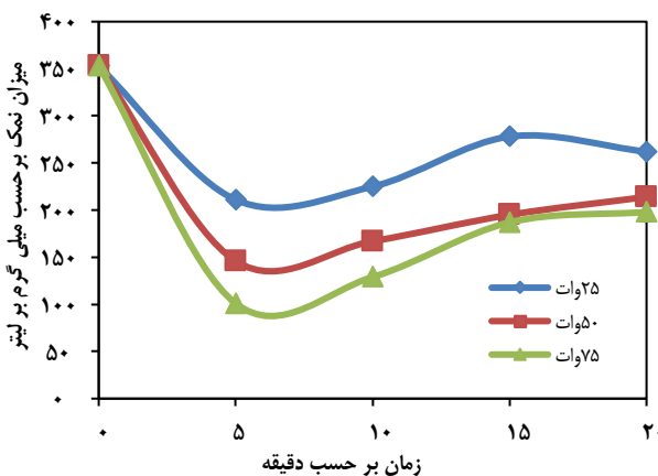
شکل ۱۳- میزان نمک اهواز ۴ با توان‌های ورودی (۲۵، ۵۰ و ۷۵) با زمان‌های تابش متفاوت در میدان موج ایستاده با فرکانس ۲۰ kHz، زمان ته نشینی ۶۰ دقیقه و تزریق ۵٪ آب شست و شو و ۳۰ ppm تعلیق شکن در دمای ۸۰ درجه سلسیوس
