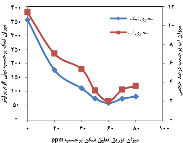
شکل ۴- تأثیر تزریق تعلیق شکن بر نمک‌زدایی و آب‌زدایی از نمونه نفت اهواز ۴
