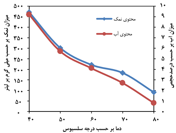
شکل ۷- میزان نمک نمونه نفت اهواز ۱ در دماهای گوناگون تزیق ۲۰ kHz و ۵٪ آب شست و شو و ۴۰ ppm تعلیق شکن تابش فراصوت با قدرت ۷۵ W و زمان ۶۰ دقیقه
