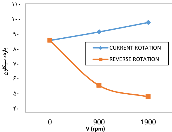
شکل ۷- نمودارهای مربوط به اثر سرعت در راستای جریان و وارون جریان در شدت جریان ۷۰ متر مکعب بر ساعت و با پودرهای ۴۰ میکرونی
