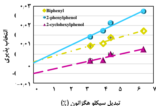
شکل ۵ - انتخاب پذیری برای تشکیل فراورده‌های به دست آمده در تبدیل سیکلو هگزانون کاتالیز شده با \text{Pt}/\gamma\text{Al}_2\text{O}_3 در حضور گاز هیدروژن در T=673\text{K} و P=14\text{bar} .
