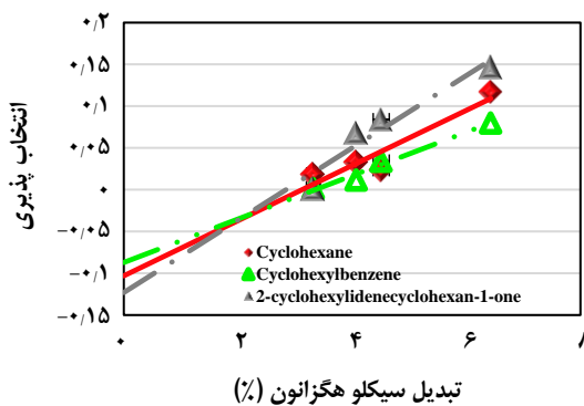
شکل ۵ - انتخاب پذیری برای تشکیل فراورده‌های به دست آمده در تبدیل سیکلو هگزانون کاتالیز شده با \text{Pt}/\gamma\text{Al}_2\text{O}_3 در حضور گاز هیدروژن در T=673\text{K} و P=14\text{bar} .
