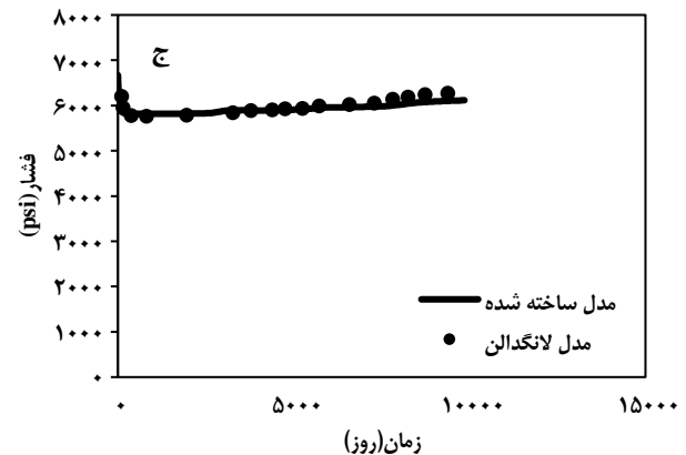
شکل ۵ نمودار کل نفت تولیدی (الف)، برش آب (ب) و فشار مخزن (ج) بر حسب زمان، (۴]۰)
