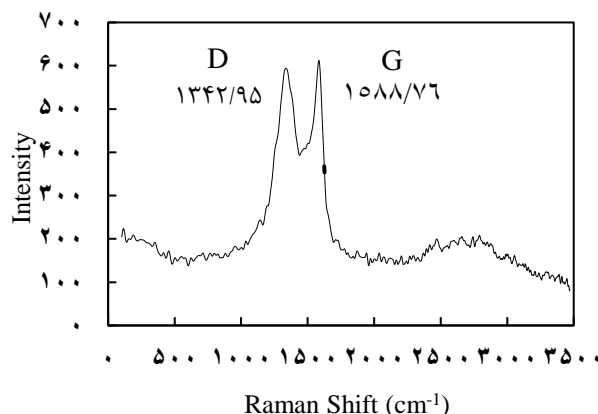
شکل ۳ - طیف رامان گرافن اکسید سنتز شده با روش MGO
