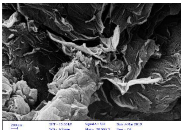
شکل ۵ - تصویری از گرافن اکسید توسط میکروسکوپ الکترونی روبشی با ۲۰۰ برابر بزرگنمایی
