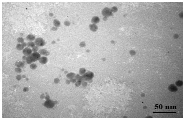
شکل ۵ - تصاویرهای TEM نانوذره‌های نقره/نقره کلرید سنتز شده با میوه جم
