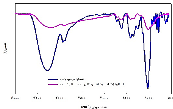
شکل ۶ - طیف FT-IR عصاره میوه گیاه جم و نانوذره‌های نقره/نقره کلرید سنتز شده
