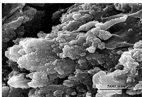
شکل ۳ - تصویر FESEM نانوذره‌های نقره/نقره کلرید با استفاده از میوه گیاه جم
