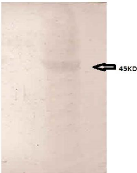
شکل ۶. تست لکه گذاری وسترن پروتئین FSH نو ترکیب
