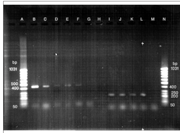
تصویر ۱- تصویر از ژل آگارز ۱/۷ درصد. ستون های A و N مارکر DNA 50bp، تصویر مثبت کنترل استافیلوکوکوس اورئوس (استخراج DNA به وسیله کیت)، C کنترل مثبت استافیلوکوکوس اورئوس (استخراج DNA به وسیله جوشاندن)، D تا G نمونه های تکثیر شده با استفاده از پرایمرهای Uni1870 و Uni2308، H کنترل منفی و I تا M نمونه های تکثیر شده با استفاده از پرایمرهای Uni678 و Uni888 را نشان می دهند.
