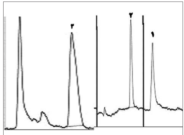
نمودار ۱- دو نمونه از کروماتوگرام‌های کلوزانتل که در آن، ۱= بلانک، ۲= استاندارد و ۳= سرم استخراج شده از خون یکی از گوسفندان تحت مطالعه را نشان می‌دهد.
