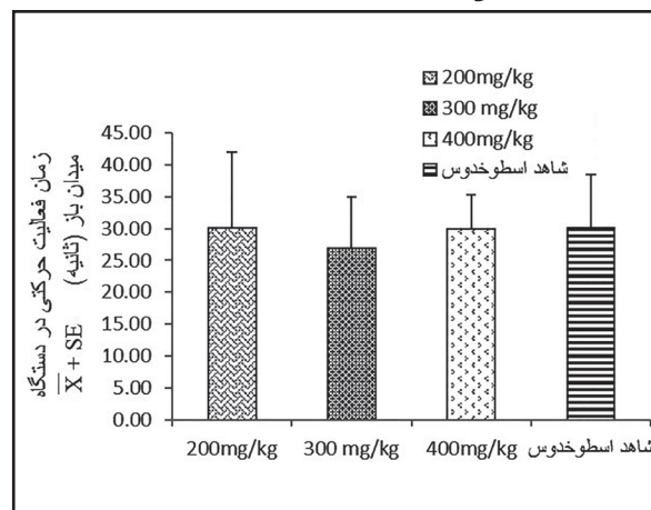
نمودار ۳. مقایسه میانگین زمانی مربوط به میزان فعالیت حرکتی در دستگاه میدان باز بین گروه شاهد و گروه‌های دریافت کننده عصاره اسطوخدوس (Locomotion time in open field) زمان فعالیت حرکتی در دستگاه میدان باز.
