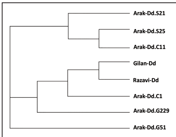
تصویر ۱. درخت فیلوژنتیک ایزوله‌های گاو، گوسفند و بز دیکروسلیوم دندردیتیکوم جمع آوری شده از کشتارگاه استان مرکزی براساس ناحیه ND1 (mtDNA) و استفاده از الگوریتم neighbor joining با ۲۰۰۰ بازتکرار در استان مرکزی.
