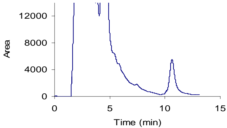
شکل ۵- کروماتوگرام لاپاکول استخراج شده با روش متانول سرد
