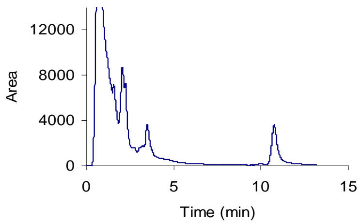
شکل ۶- کروماتوگرام لاپاکول استخراج شده با روش آب داغ
