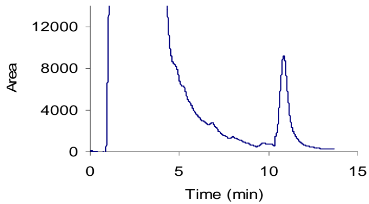
شکل ۴- کروماتوگرام لاپاکول استخراج شده با روش متانول گرم شده در مایکروویو
