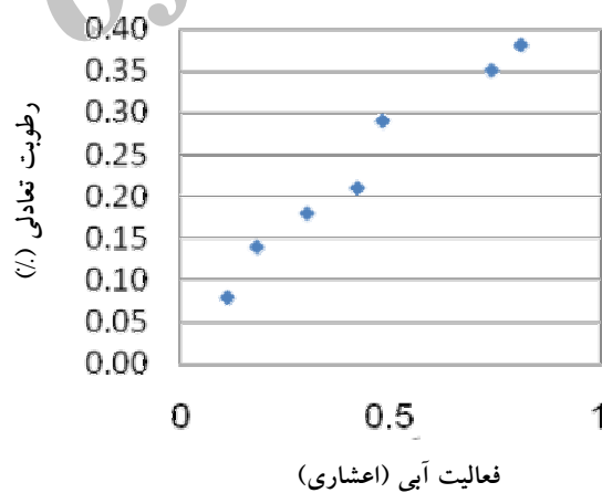
شکل ۲- مقادیر رطوبت تعادلی در اثر تغییرات رطوبت نسبی محیط در دمای 50^{\circ}\text{C} برای پدیده جذب (بدون بارش)
