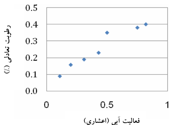
شکل ۱- مقادیر رطوبت تعادلی در اثر تغییرات رطوبت نسبی محیط در دمای 40^{\circ}\text{C} برای پدیده جذب (بدون بارش)
