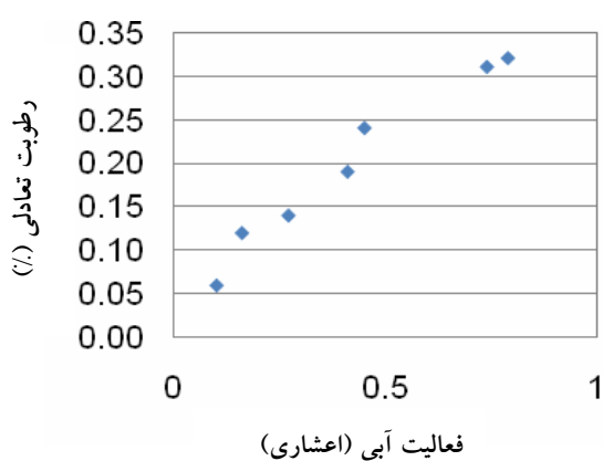
شکل ۴- مقادیر رطوبت تعادلی در اثر تغییرات رطوبت نسبی محیط در دمای 70^{\circ}\text{C} برای پدیده جذب (بدون بارش)
