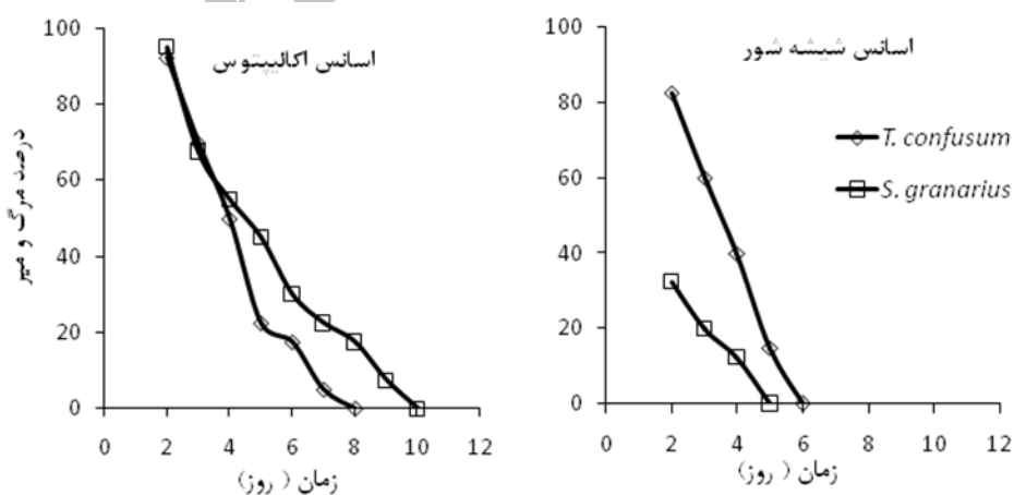
شکل ۲- دوام اسانس اکالیپتوس و شیشه شور بعد از گذشت روزهای مختلف روی شیشه آرد و شیشه گندم
